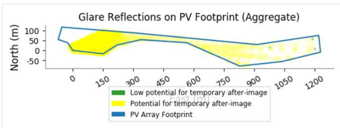
Abbildung 20: PV-Anlage B: Fläche mit Reflexionen auf OP2
