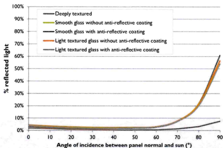
Abbildung 10: Reflexionseigenschaften typischer Abdeckgläser (Quelle: (Yamada T.))
