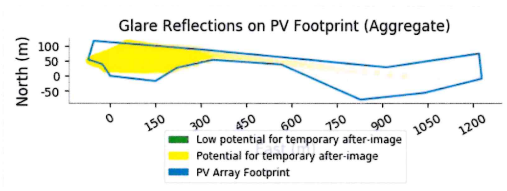
Abbildung 17: PV-Anlage B: Fläche mit Reflexionen auf OP1
