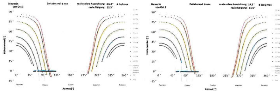
Abbildung 13: Reflexionsdiagramme für Punkt 1 der Bahnlinie aus Osten, links für die minimal auftretende Ausrichtung, rechts für die maximale
