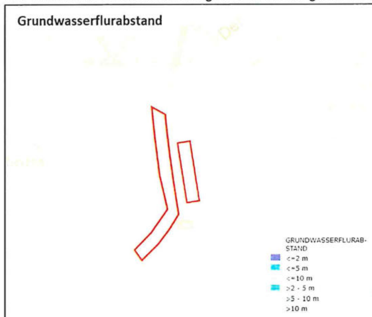
Abbildung 5 Grundwasserflurabstand
