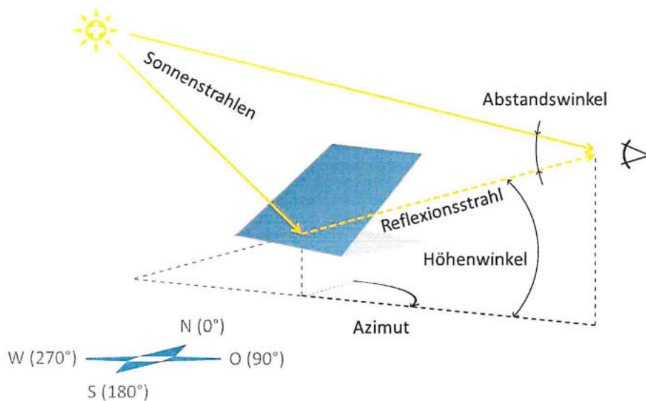
Abbildung 7: Darstellung des Reflexionsstrahls anhand von Azimut und Höhenwinkel wie im Reflexionsdiagramm verwendet und Beschreibung des Abstandswinkels zwischen Blickrichtungen zur Sonne und zum Blendpunkt
