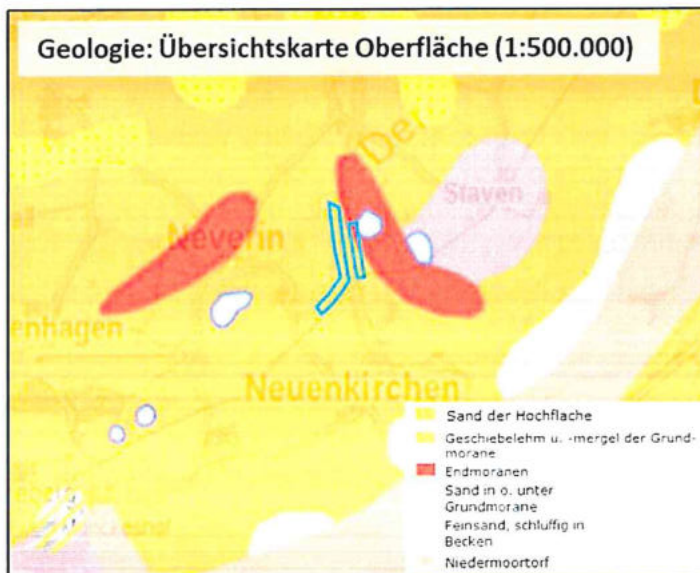
Abbildung 6 Übersichtskarte Geologie
