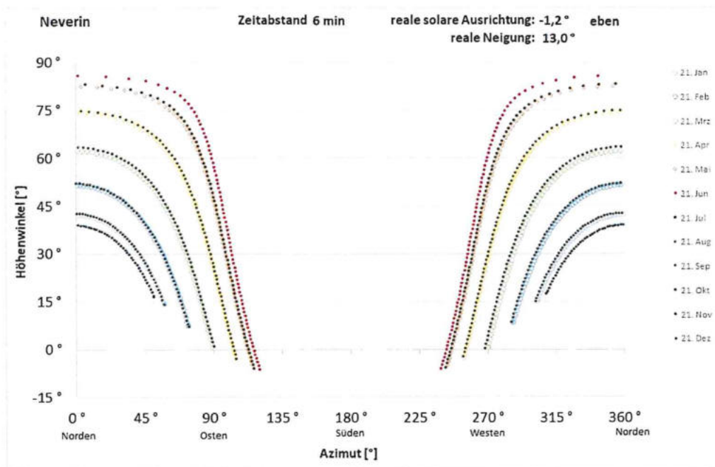
Abbildung 8: Reflexionsdiagramm aus Sicht eines beliebigen potenziellen Blendpunktes eines Modultisches auf ebenem Grund mit einer Ausrichtung von -1,2^\circ und einer Modulneigung von 13,0^\circ am Standort der Anlage; waagrecht aufgetragen sind die Azimutwinkel von Norden ( 0^\circ ) über Osten ( 90^\circ ), Süden ( 180^\circ ) nach Westen ( 270^\circ ), senkrecht die Höhenwinkel
