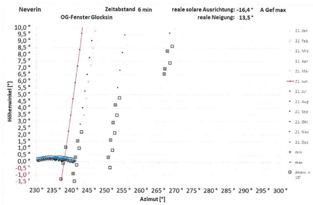
Abbildung 20: Detailausschnitt des linken Diagramms aus Abbildung 19; Reflexionen mit Abständen zur Sonne von unter 10°, die nach LAI-Richtlinie nicht als Immissionen gewertet werden, sind schwarz umrahmt
