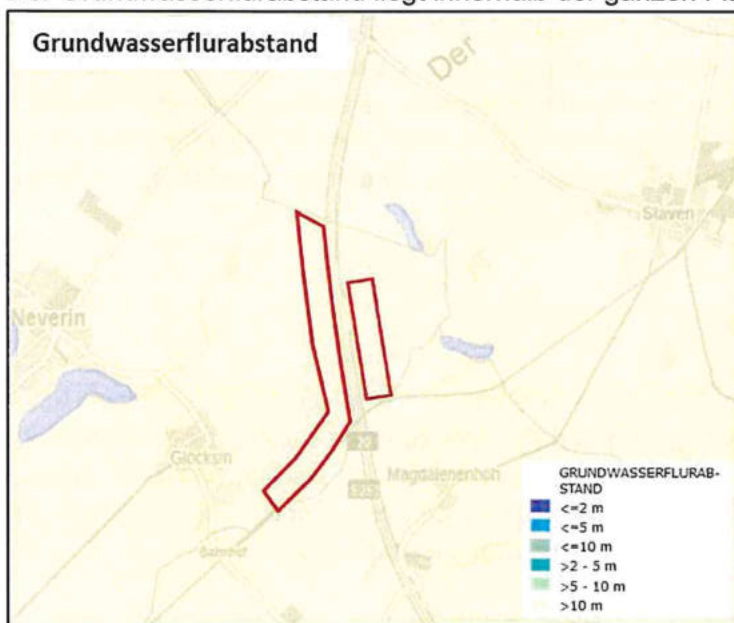
Abbildung 8 Grundwasserflurabstand
